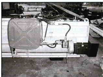
Ekstraudstyr Hydraulisk Power pack 32 L/min eller 60 L/min.
